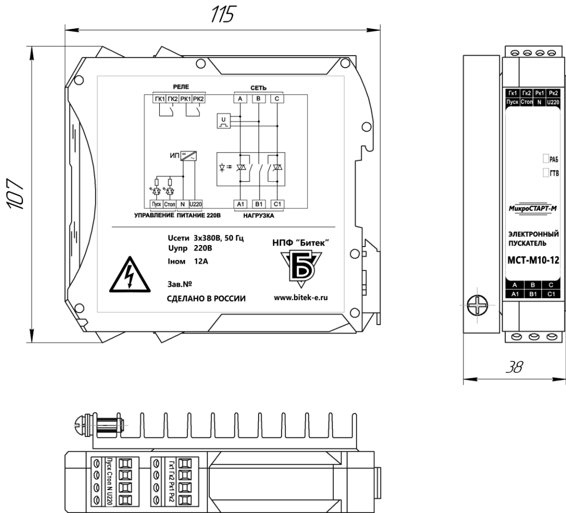
Рисунок А.2 – Габаритно-установочные размеры МСТ-1х-12
