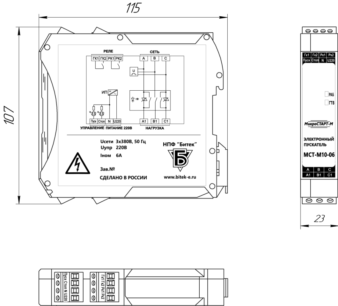
Рисунок А.1 – Габаритно-установочные размеры МСТ-М1х-03, МСТ-М1х-06
