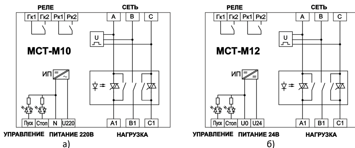
Рисунок 2 – Функциональная схема пускателей а) МСТ-М10-хх, б) МСТ-М12-хх
