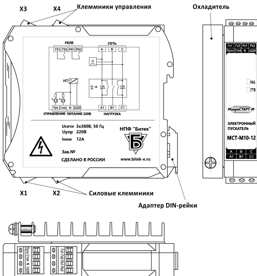
Рисунок 1 - Внешний вид блока МСТ-М10-12
