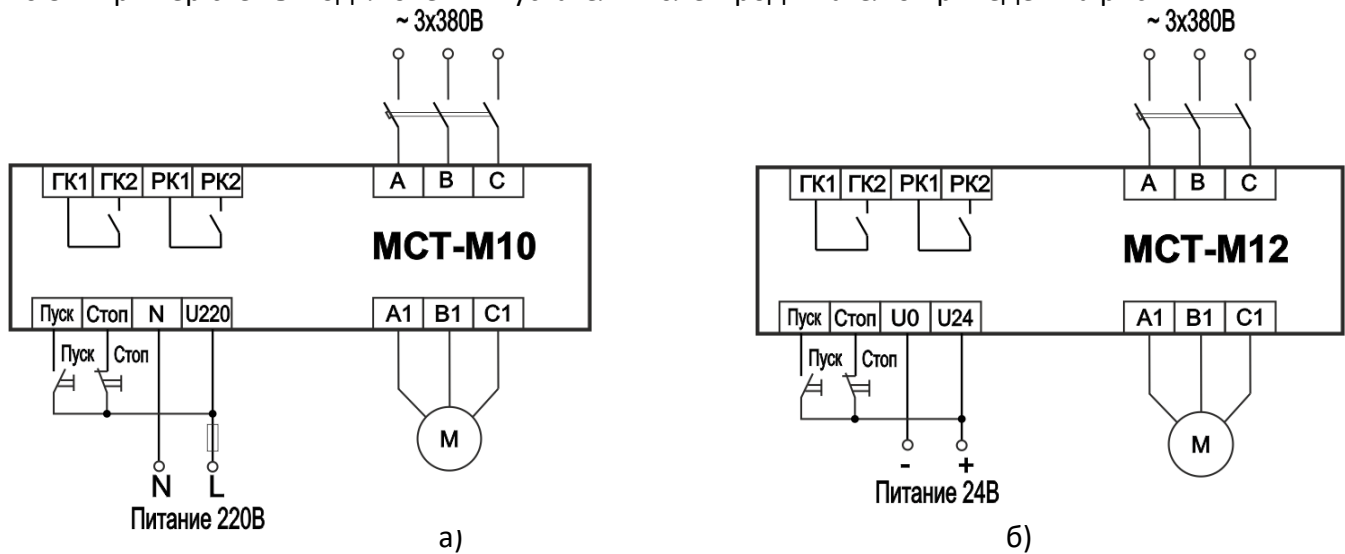
Рисунок 4 – Пример схемы подключения пускателя а) МСТ-М10-хх, б) МСТ-М12-хх
